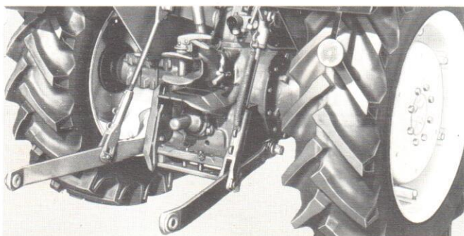
Onafhankelijk van de koppeling werkende hydraulische combinatieregeling via de onderste trekstangen.
