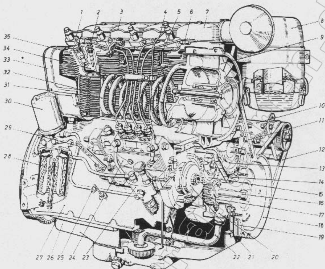
Schnittbild F 4 L 812
