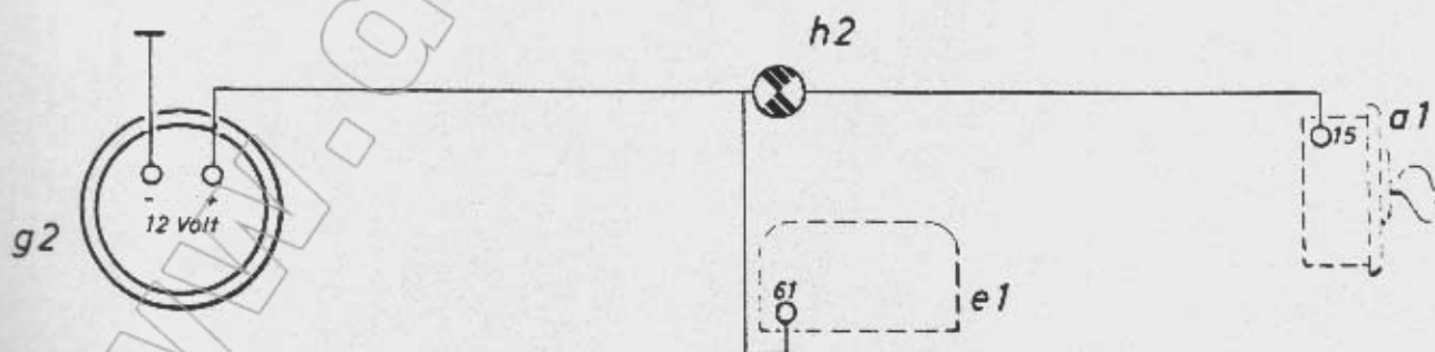
Schaltplan Betriebsstundenzähler
