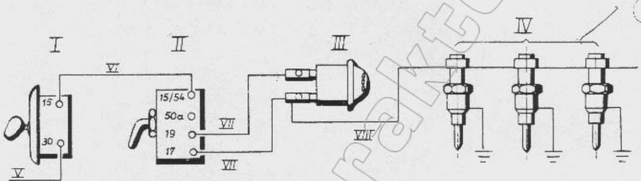
Schema einer F 3 L 812-Glühstiftanlage
