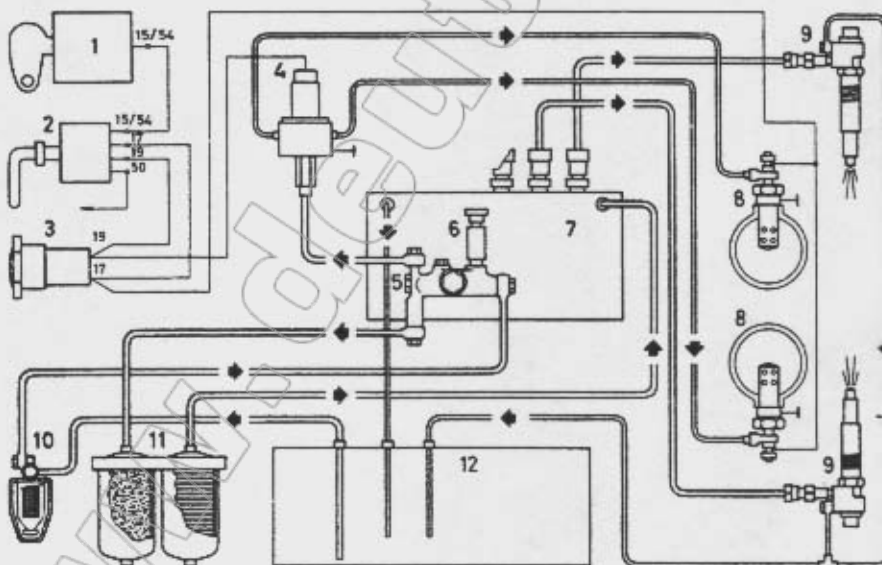
Schema der Kraftstoffanlage und Anordnung der Flammglühkerzen
