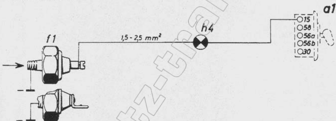
Schaltplan Öldruckwarnanlage 12 oder 24 Volt
