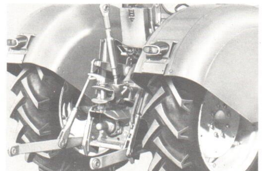
Onafhankelijk van de koppeling werkende hydraulische 3-punts hefinrichting met automatische regeling via de onderste trekstangen.
